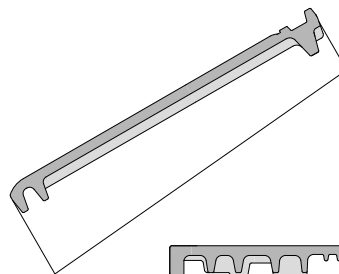
Ortgangziegel links Querschnitt
