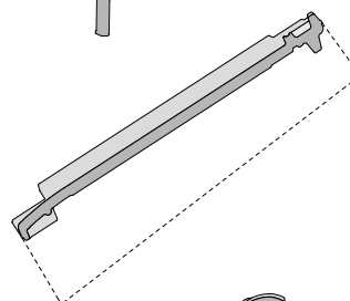
Ortgangziegel rechts Längsschnitt
